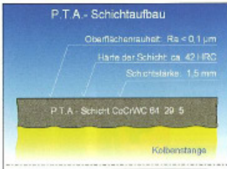
Aufbau einer P.T.A.-Schicht.
